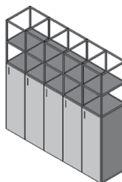
L/W237 P/D60 H237
