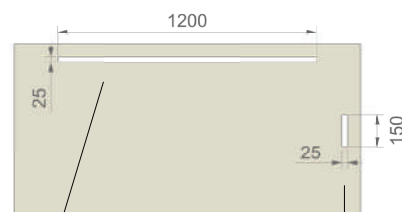
PASSE-CÂBLES - PORTE ACCESSOIRES
