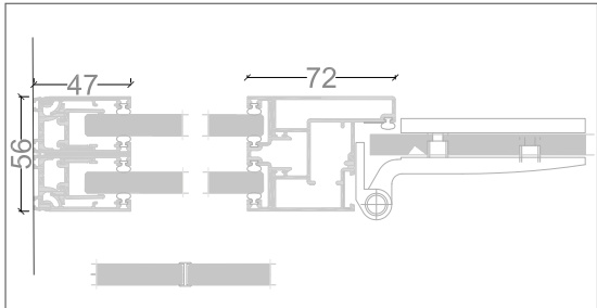
HORIZONTAL SECTION GLASS DOOR
