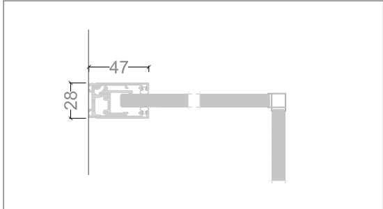
90° ANGLE
