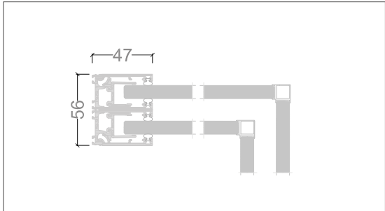
90° ANGLE
