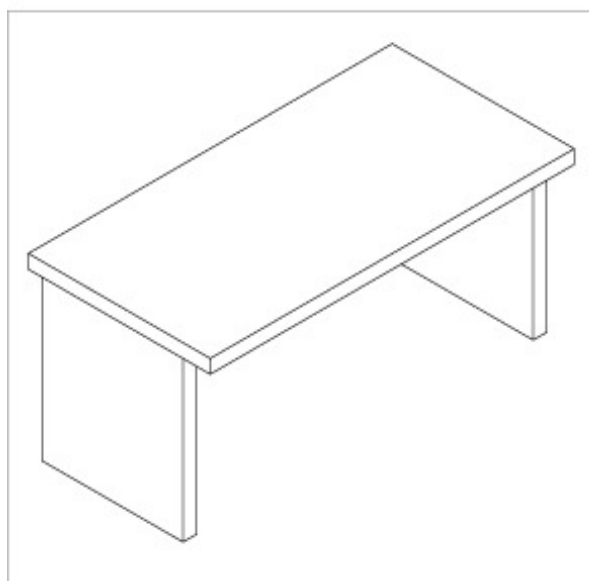
SCHEMA DI MONTAGGIO DELLE SCRIVANIE PANNELLATE
