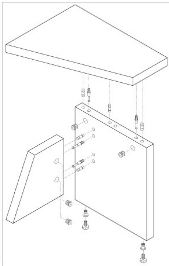
SCHEMA DI MONTAGGIO DELLE SCRIVANIE PANNELLATE
