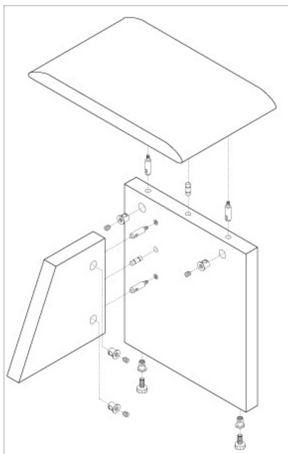
SCHEMA DI MONTAGGIO SCRIVANIE PANNELLATE NEW ROSSANA
