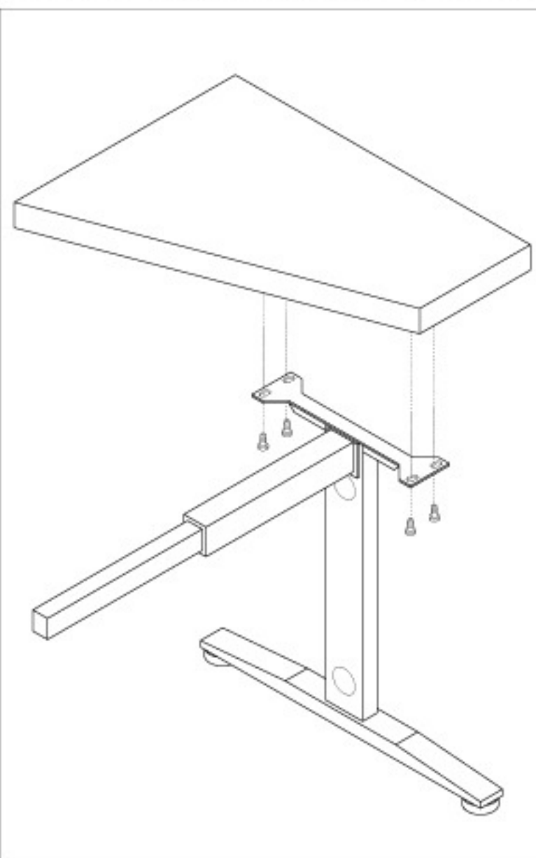
SCHEMA DI MONTAGGIO DELLE SCRIVANIE METALLICHE
